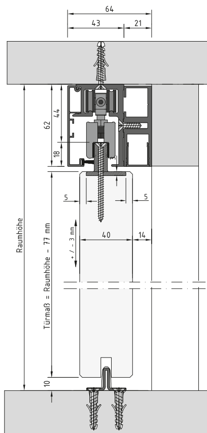
Montage vor Sturz mit Holztür
