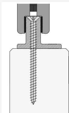
L&H T-Profil aufgesetzt und verschraubt
